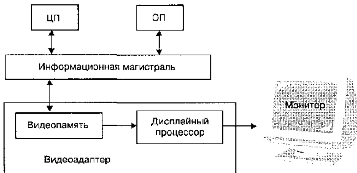
Рис. 4.7. Схема системы вывода изображения на экран.
